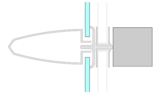
図15 クリシーの人民の家(1938)： カーテンウォールの外壁[左]と断面図解図[右] ④
