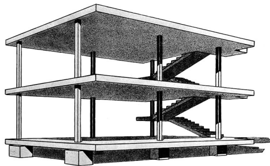
図7 ル・コルビュジェによる「ドミノ」の理論と実践 ⑫
